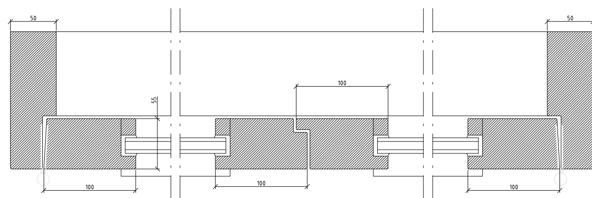
DETALJ HORIZONTALSNITT
