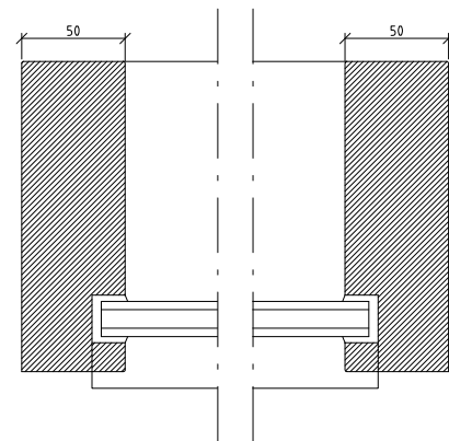
DETALJ HORIZONTALSNITT
