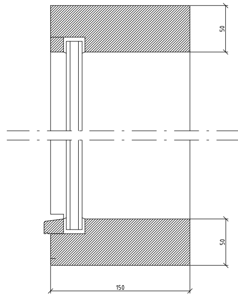
DETALJ VERTIKALSNITT
