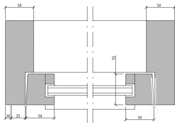
DETALJ HORIZONTALSNITT
