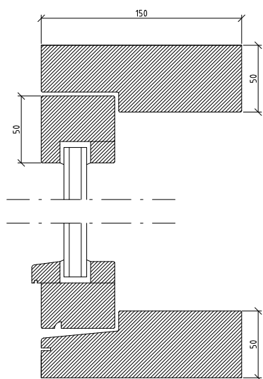
DETALJ VERTIKALSNITT
