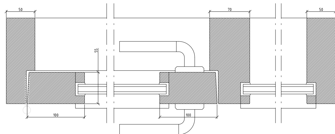
DETALJ HORIZONTALSNITT
