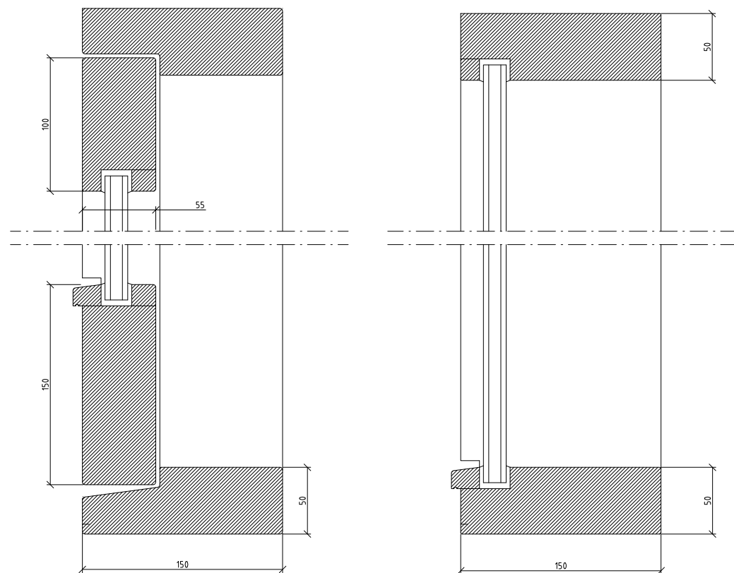
DETALJ VERTIKALSNITT
